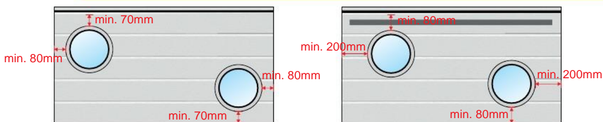
Ukse laius L \leq 4500 mm
